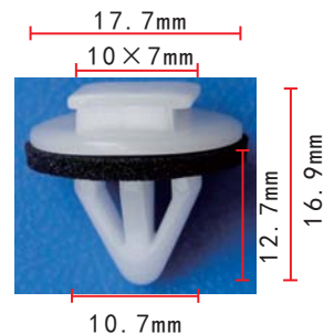
C1478 POM White Door Moulding Clip
