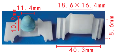
C908 POM White Side Moulding Grommet VW & Audi
