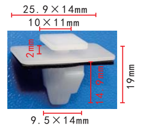
C987 POM White Nut Hyundai, Kia
