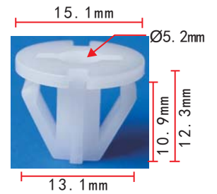
C987 POM White Nut Hyundai, Kia
