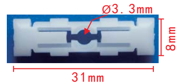
C915 POM White Door Moulding Clip VW & Audi
