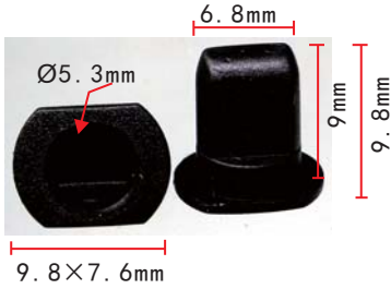
C1575 Nylon Black Retainer VW Jetta 171-853-615A, 191853615A
