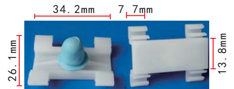
C903 POM White Door Shield Moulding Clip Mercedes-Benz 124 & 201
