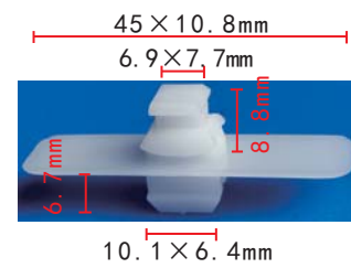
C974 POM White Retainer Mercedes-Benz 0069888978
