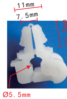
C367 Nylon White Door Lock Rod End Clip Mazda E6DZ5421952A E83Z-5421952
