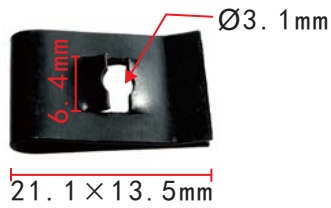
H2006 Nut vw
