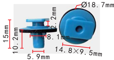
C3223 POM Blue Door Trim Clip Nissan#90990-1KA0B
