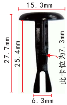
C962 POM Black Retainer
