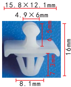
C979 POM White Retainer Mercedes-Benz 0019884481
